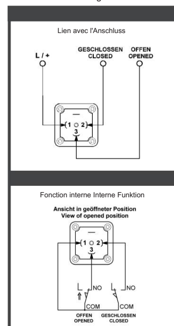
Buchsen de position finale Endlagenstecker
